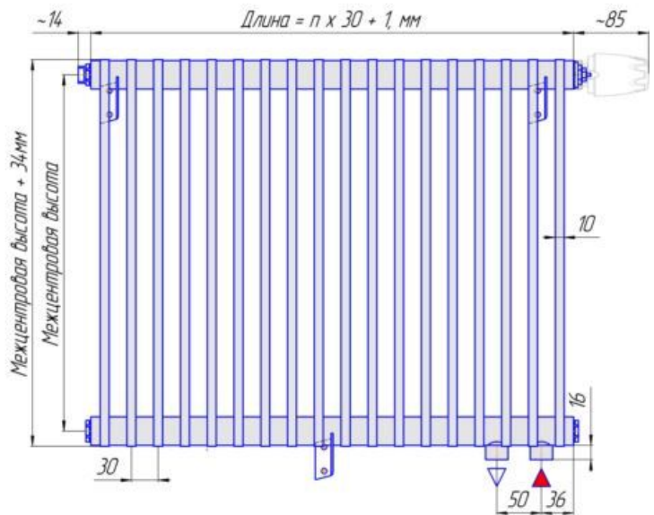
Присоединительная резьба G 1/2" внутр.
