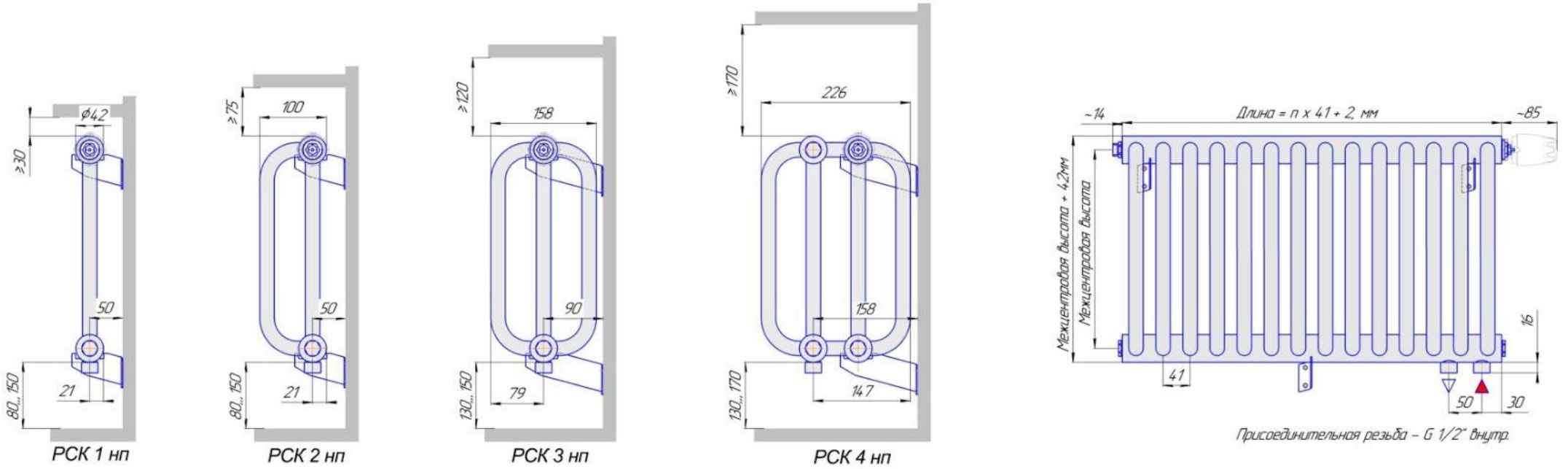
Радиаторы "РСК нп", монтажные схемы
