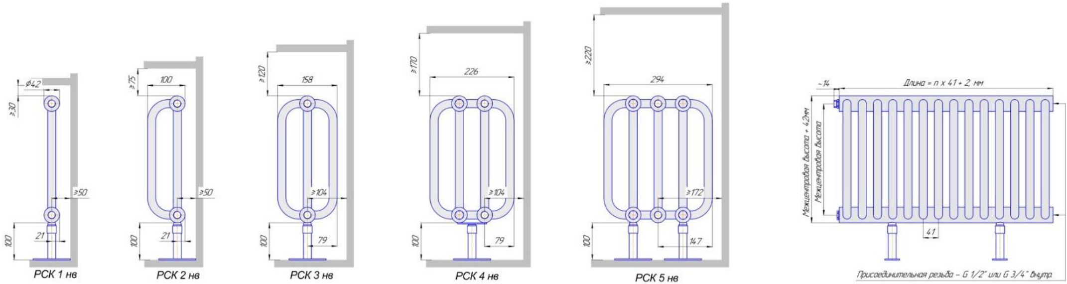
Радиаторы "РСК нв", монтажные схемы
