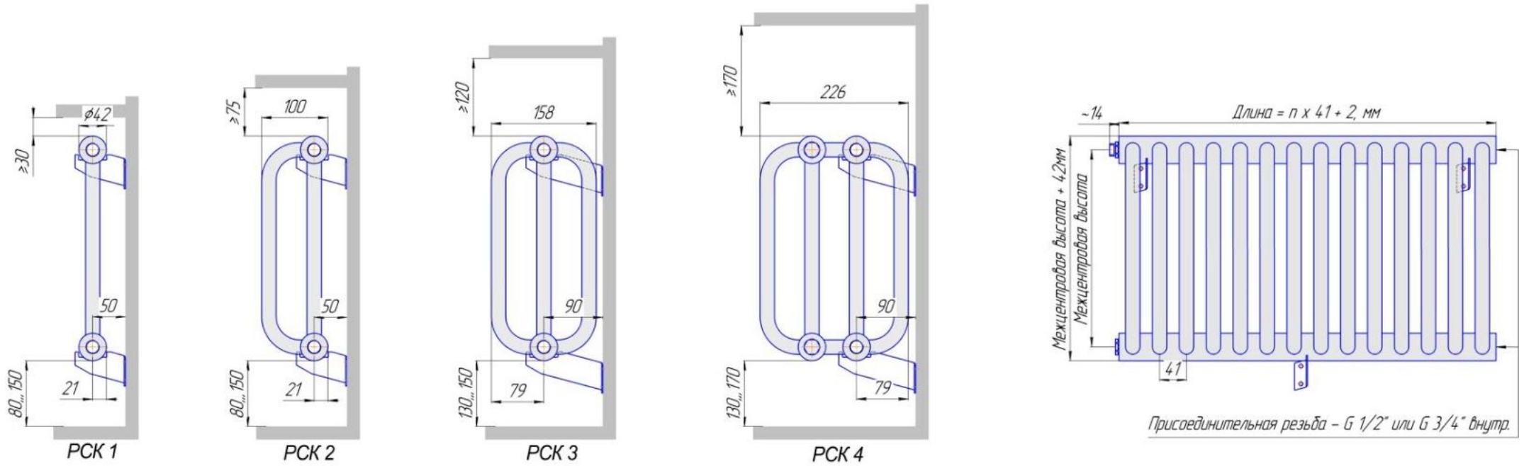
Радиаторы "РСК", монтажные схемы
