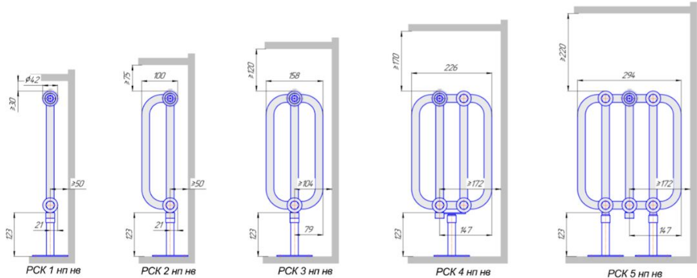
Радиаторы "РСК нп нв", монтажные схемы
