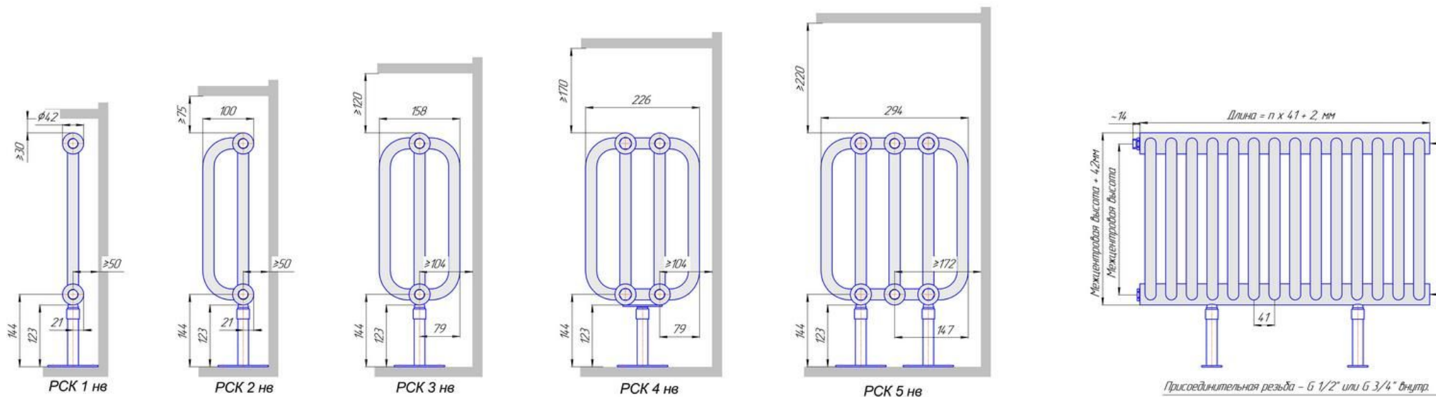
Радиаторы "РСК нв", монтажные схемы
