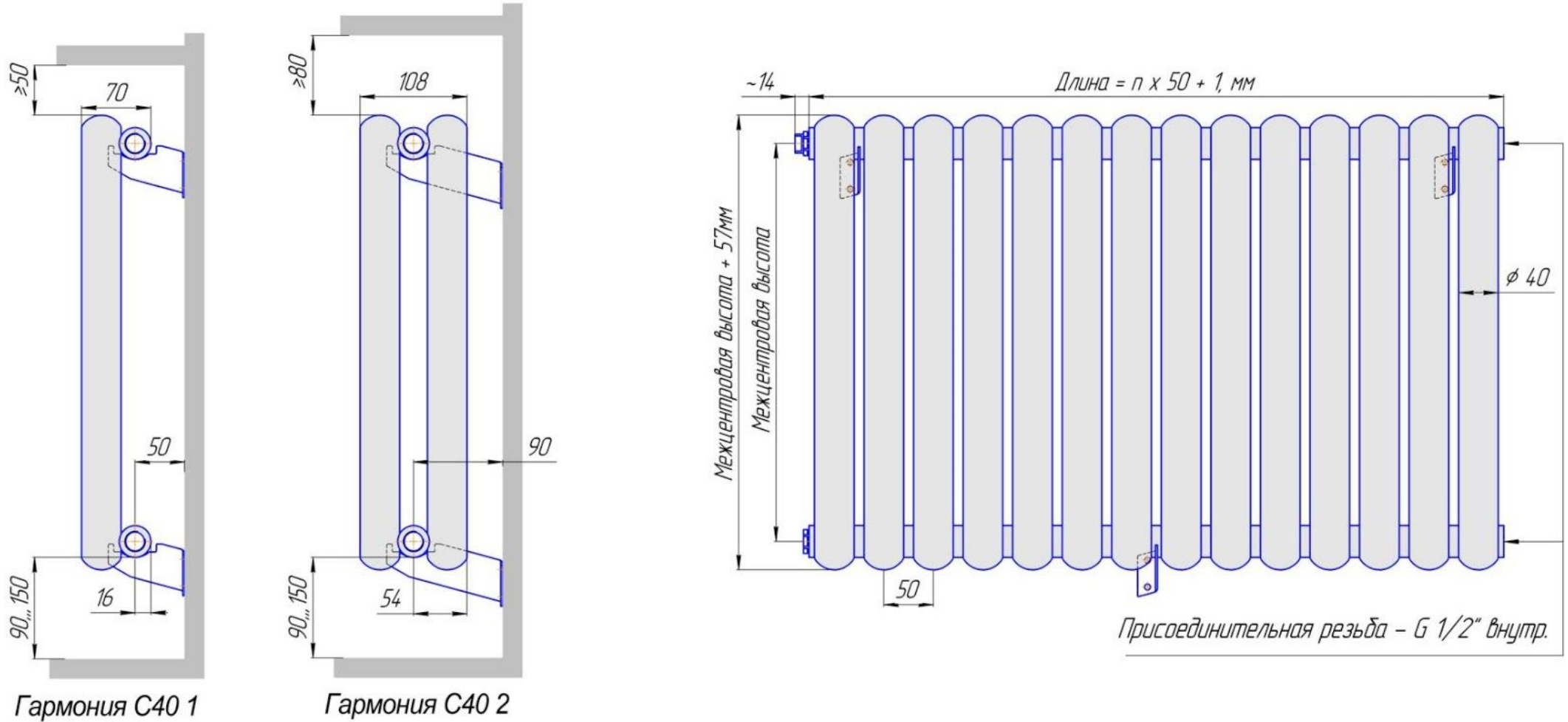
Радиатор Гармония С40, монтажная схема
