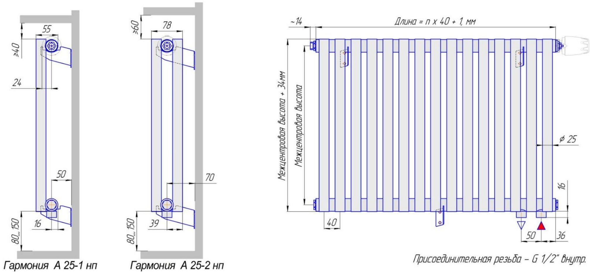
Радиатор "Гармония А25 нп", монтажная схема
