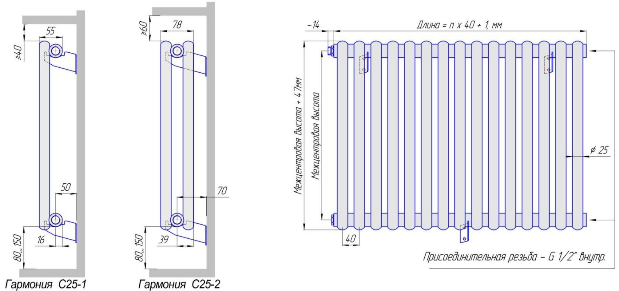
Радиатор "Гармония С25", монтажная схема
